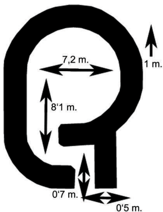
M.G.P. 001. Planta i mesures. Casamata les Deveses II.
